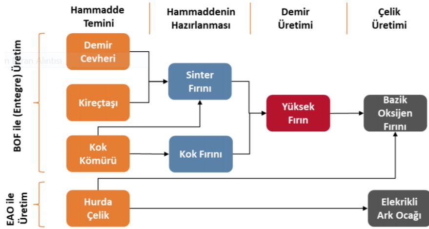
Şekil 1.1. Üretim Yöntemlerine Göre Çelik Üretimi
