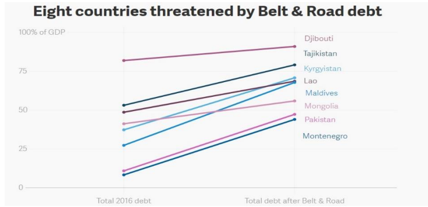
Resim 2. OBOR borçları nedeniyle tehdit altında bulunan sekiz ülke.
